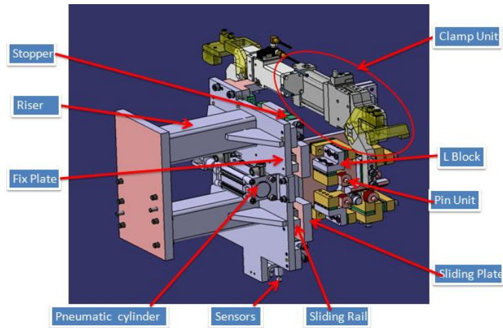
Fig. 5: Slide Unit.
