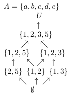
mL(U, A, F)
